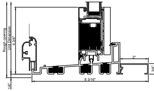
6 9/16" Std. Sill
